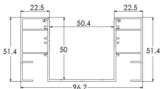
ZSS323 - CON DOPPIO DISTANZIALE DA 23
