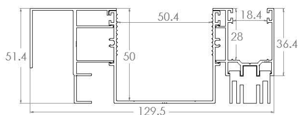
ZSS323 - GUIDA LARGA E DISTANZIALE DA 46
