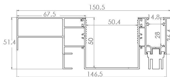
ZSS323 - GUIDA MINI CON ALETTA E DISTANZIALE DA 68
