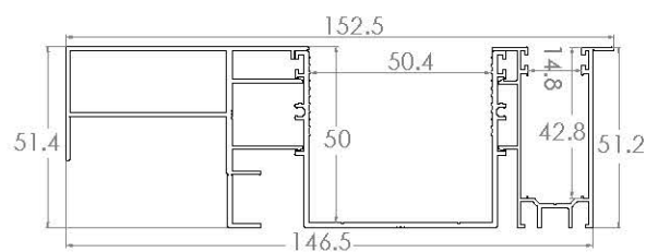
ZSS323 GUIDA PROFONDA MINI CON ALETTA E DISTANZIALE DA 68
