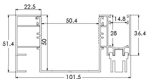
ZSS323 - GUIDA MINI E DISTANZIALE DA 23
