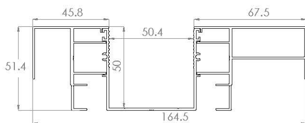
ZSS323 - DISTANZIALE DA 46 E DA 68
