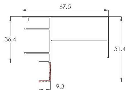
ZAP352 DISTANZIALE DA 68
