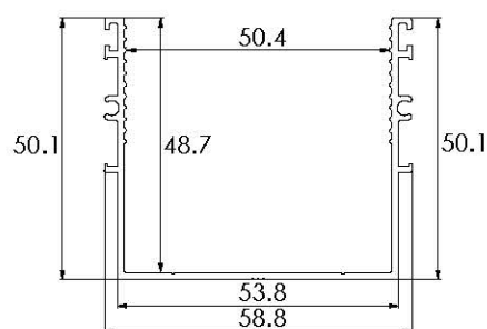
ZAP312 PREDISPOSIZIONE 50x50 AGGANCIAMENTO BILATERALE
