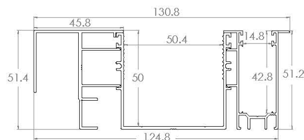
ZSS323 GUIDA PROFONDA MINI CON ALETTA E DISTANZIALE DA 46
