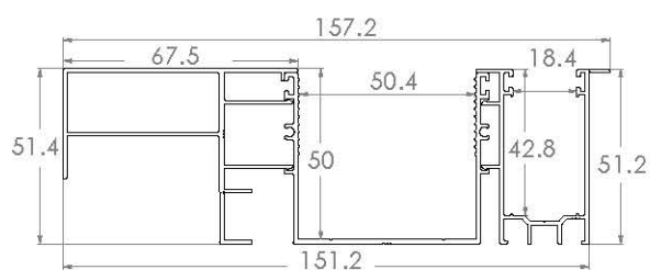
ZSS323 - GUIDA PROFONDA LARGA CON ALETTA E DISTANZIALE DA 68
