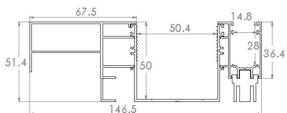
ZSS323 - GUIDA MINI E DISTANZIALE DA 68
