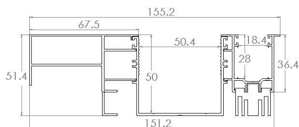
ZSS323 - GUIDA LARGA CON ALETTA E DISTANZIALE DA 68
