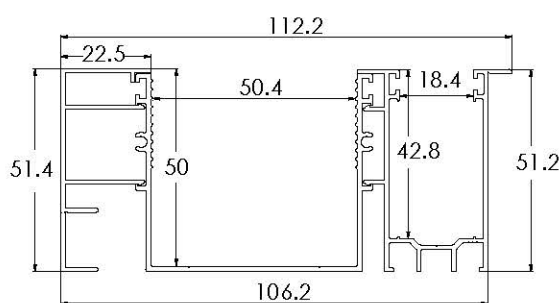
ZSS323 - GUIDA PROFONDA LARGA CON ALETTA E DISTANZIALE DA 23
