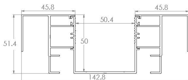
ZSS323 - CON DOPPIO DISTANZIALE DA 46
