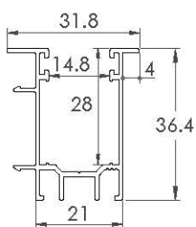
ZAP341 GUIDA MINI con aletta
