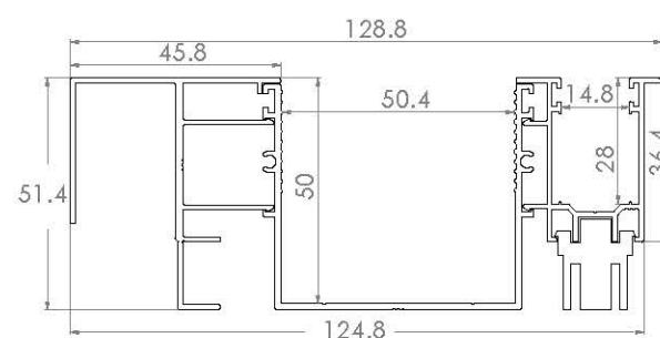
ZSS323 - GUIDA MINI CON ALETTA E DISTANZIALE DA 46
