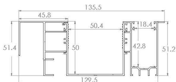
ZSS323 - GUIDA PROFONDA LARGA CON ALETTA E DISTANZIALE DA 46
