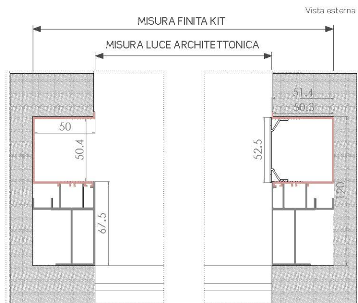
SEZIONE ORIZZONTALE
