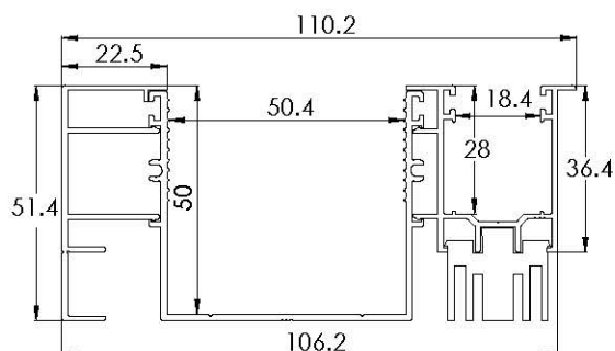
ZSS323 - GUIDA LARGA CON ALETTA E DISTANZIALE DA 23
