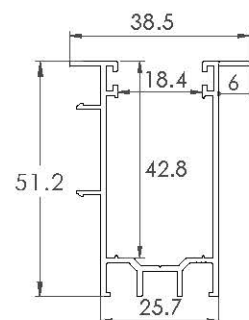
ZAP332* GUIDA PROFONDA con aletta
