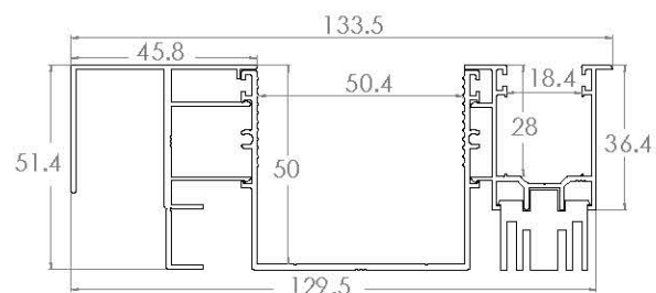
ZSS323 - GUIDA LARGA CON ALETTA E DISTANZIALE DA 46
