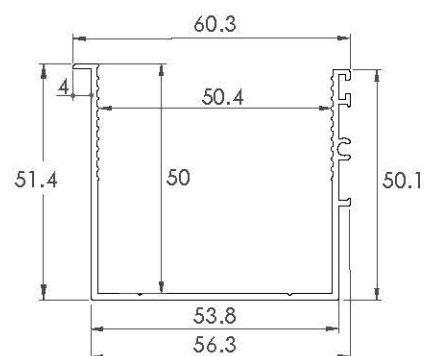
ZAP311 PREDISPOSIZIONE 50x50 CON ALETTA
