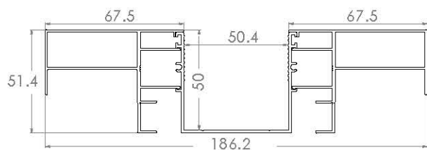
ZSS323 - CON DOPPIO DISTANZIALE DA 68
