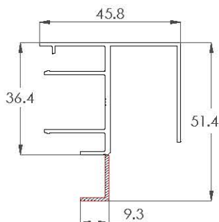
ZAP351 DISTANZIALE DA 46
