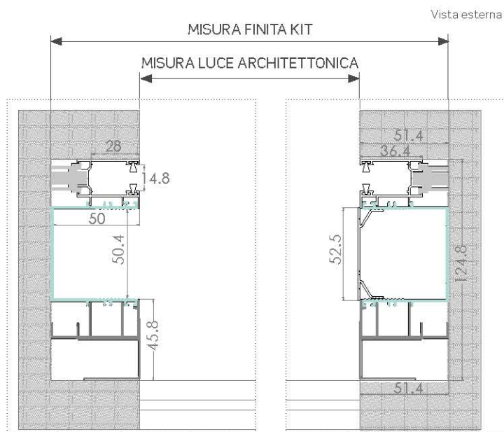
SEZIONE ORIZZONTALE Vista interna
