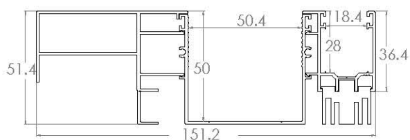
ZSS323 - GUIDA LARGA E DISTANZIALE DA 68
