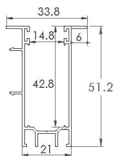
ZAP342* GUIDA PROFONDA MINI con aletta
