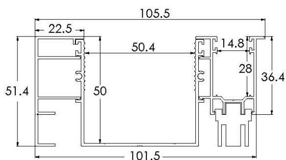
ZSS323 - GUIDA MINI CON ALETTA E DISTANZIALE DA 23
