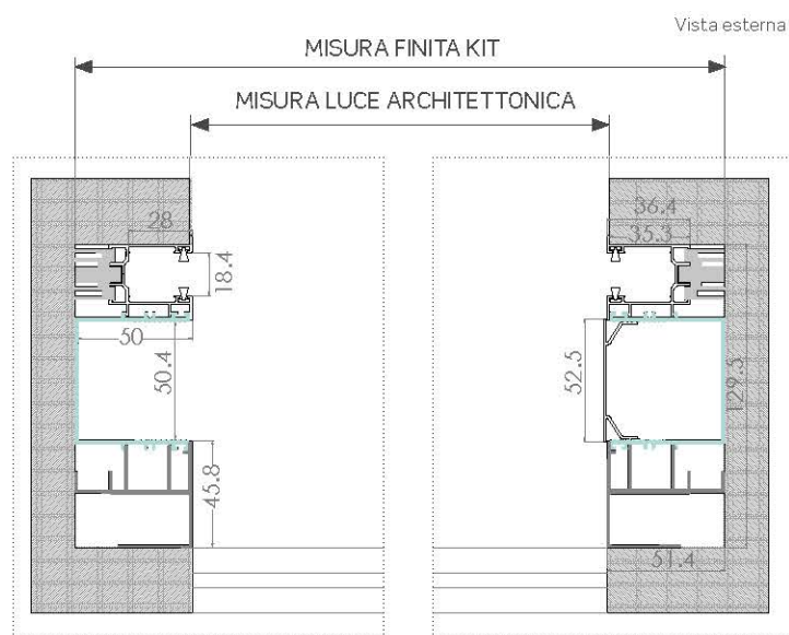
SEZIONE ORIZZONTALE Vista esterna Vista interna
