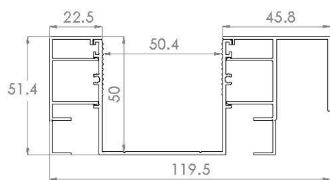
ZSS323 - DISTANZIALE DA 23 E DA 46
