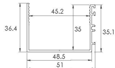
ZAP320 PREDISPOSIZIONE 45x35
