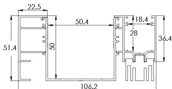
ZSS323 - GUIDA LARGA E DISTANZIALE DA 23
