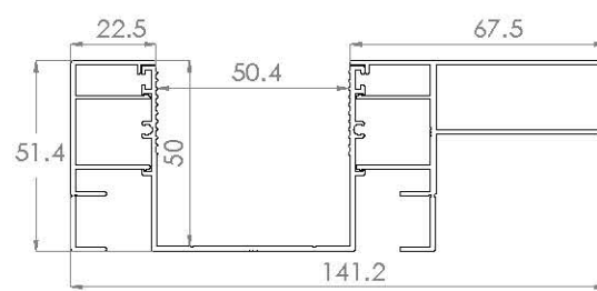
ZSS323 - DISTANZIALE DA 23 E DA 68
