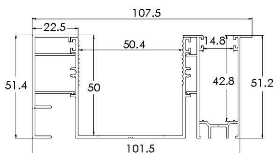
ZSS323 GUIDA PROFONDA MINI CON ALETTA E DISTANZIALE DA 23
