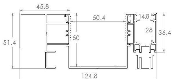
ZSS323 - GUIDA MINI E DISTANZIALE DA 46
