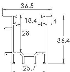
ZAP331 GUIDA LARGA con aletta
