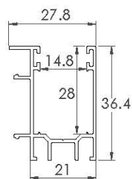
ZAP340 GUIDA MINI
