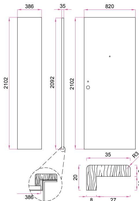
SEZIONE BATTENTE ANTA PICCOLA
