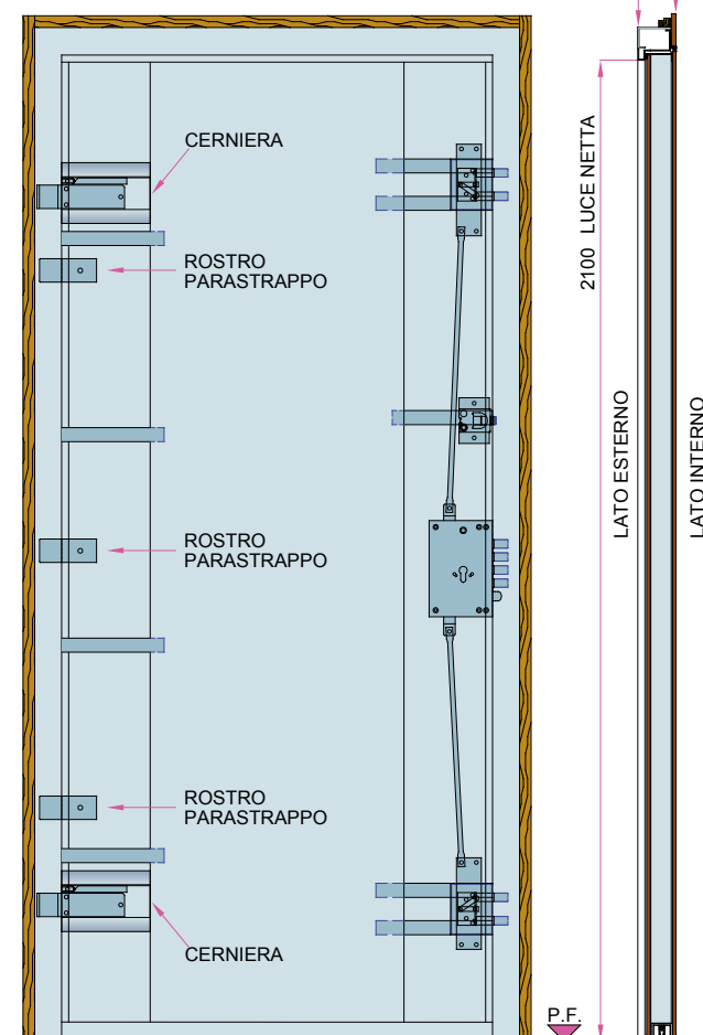
PROSPETTO lato interno e sezione verticale.
