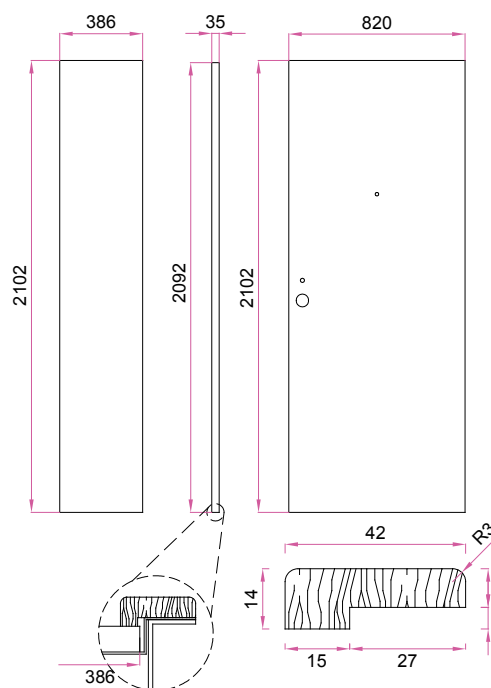
SEZIONE BATTENTE ANTA PICCOLA
