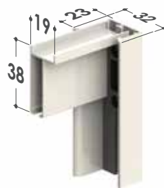
Cassonetto da 40 Testate inferiori
