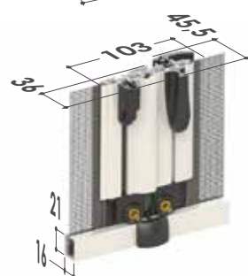
Cassonetto da 50 Testate inferiori
