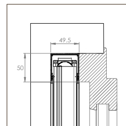
EVA INCAS MIDI 50/35
