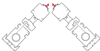
ANTA SINGOLA ANGOLARE
