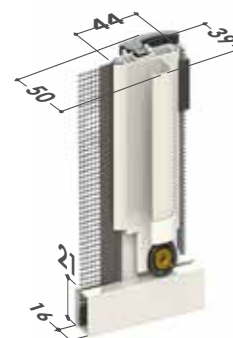
Cassonetto da 50 Testate inferiori
