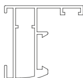
■ TELAIO AD "L"
