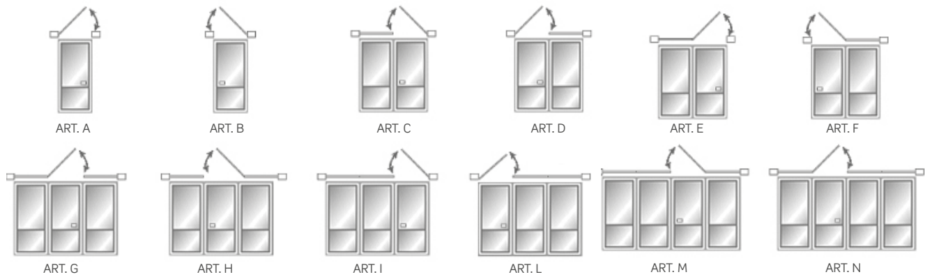
APERTURA CON VISTA INTERNA A SPINGERE
