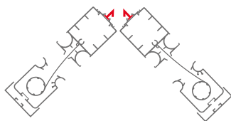
2 ANTE CON APERTURA BILATERALE ANGOLARE
