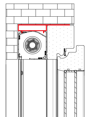
SEZIONE VERTICALE
