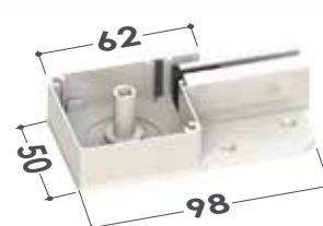
Cassonetto da 50 Testate inferiori
