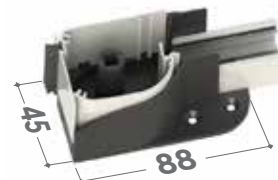
Barra maniglia singola
