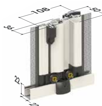
Barra maniglia doppia
