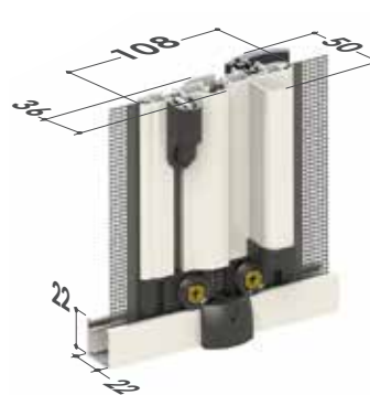
Barra maniglia doppia
