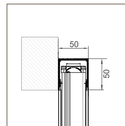
EVA UP MIDI 35/35
