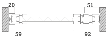
SEZIONE ORIZZONTALE 2 ANTE A SEGUIRE
