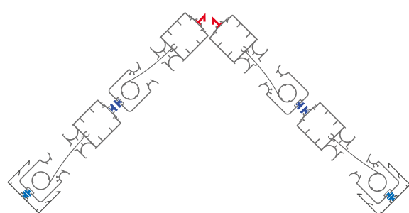
2 ANTE A SEGUIRE ANGOLARE
