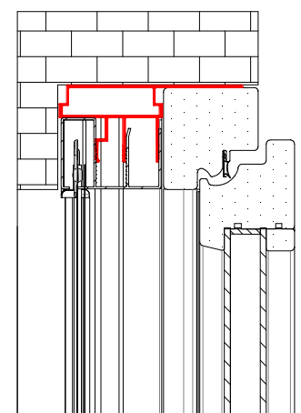
SEZIONE VERTICALE
