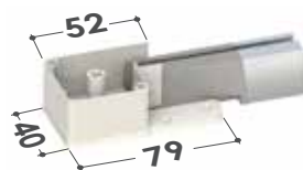
Cassonetto da 40 Testate inferiori
