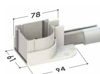
Cassonetto da 55 Testate inferiori
