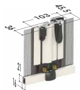
Cassonetto da 55 Testate inferiori
