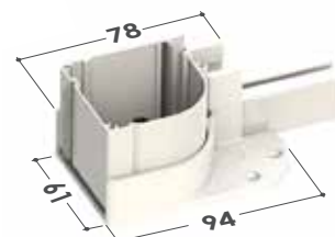
Cassonetto da 55 Testate inferiori
