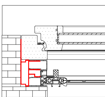
SEZIONE ORIZZONTALE
