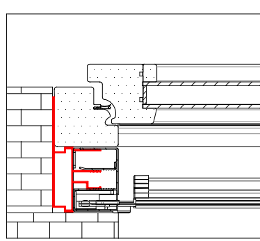
SEZIONE ORIZZONTALE
