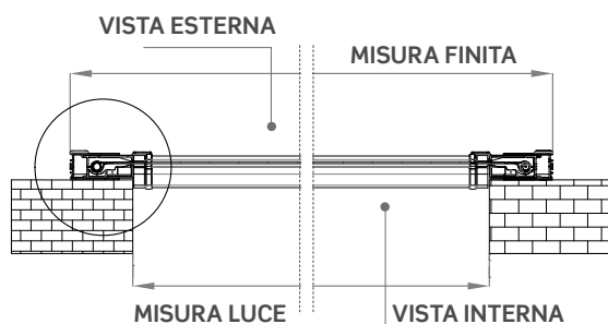
APPL. REVERSE (FIG. 2)
