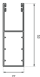
ART. Guida compatibile con mini cassonetto in alluminio
