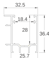
ART. ZAP 330 Profilo predisposizione con guida ad incasso per zanzariera 32,5x36,4 mm
