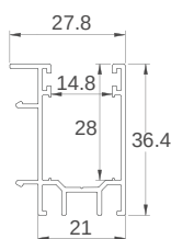
ART. ZAP 340 Profilo predisposizione con guida ad incasso per zanzariera
