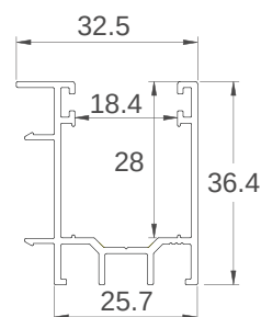
ART. ZAP 330 Profilo predisposizione con guida 32,5x36,4 mm
