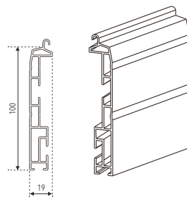
ART. Terminale in alluminio estruso
