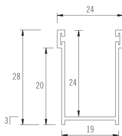
ART. 100304 Guida in alluminio estruso con spazzolino 100279
