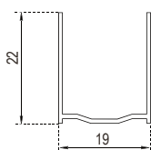
ART. 100277 Guida in ferro zincato
