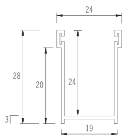
ART. 100304 Guida in alluminio estruso con spazzolino 19x28 mm
