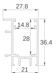
ART. ZAP 340 Profilo predisposizione con guida ad incasso per zanzariera 27,8x36,4 mm
