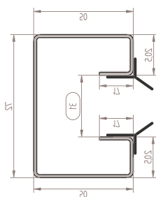
ART. Guida in alluminio per 19x77 con guarnizione
