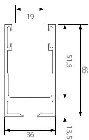
ART. 36x65 Guida in alluminio per 19x77 con guarnizione mm
