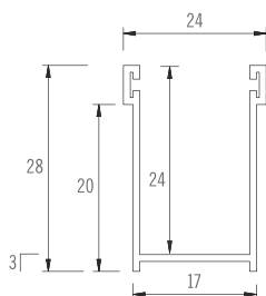
ART. 100759 Guida in alluminio estruso con spazzolino
