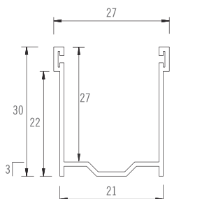
ART. 016702004 Guida in alluminio estruso con bordino e spazzolino 100279 30x27 mm
