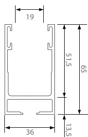
ART. Guida in alluminio per 19x77 con guarnizione
