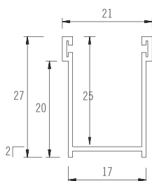
ART. 016502010 Guida in alluminio etrusco con bordino e spazzolino 100279
