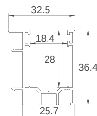
ART. ZAP 330 Profilo predisposizione con guida ad incasso per zanzariera
