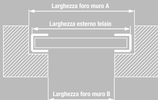
TELAIO A SPORGERE LATERALE O CENTRALE IN ALLUMINIO ROMA
