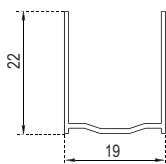
ART. 100277 Guida in ferro zincato 19x22 mm
