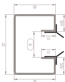
ART. 50x72 Guida in alluminio per 19x77 con guarnizione mm
