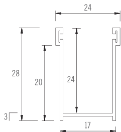
ART. 100759 Guida in alluminio estruso con spazzolino 28x17 mm
