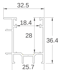
ART. ZAP 330 Profilo predisposizione con guida ad incasso per zanzariera
