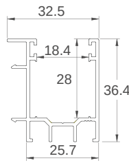
ART. ZAP 330 Profilo predisposizione con guida ad incasso per zanzariera 32,5x36,4 mm
