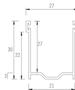
ART. 016702004 Guida in alluminio estruso con bordino e spazzolino 27x30 mm
