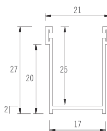
ART. 016502010 Guida in alluminio estruso con bordino e spazzolino 21x27 mm
