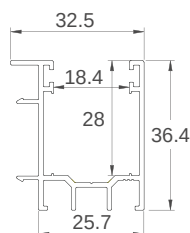
ART. ZAP 330 Profilo predisposizione con guida ad incasso per zanzariera 32,5x36,4 mm
