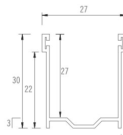
ART. 016702004 Guida in alluminio estruso con bordino e spazzolino 100279
