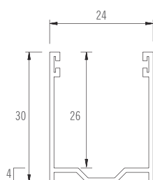
ART. 016702004 Guida in alluminio estruso senza bordino con spazzolino 24x30 mm
