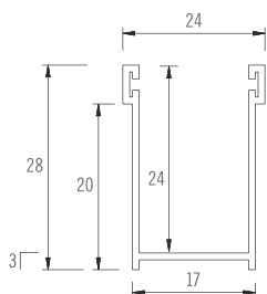
ART. 100759 Guida in alluminio estruso con spazzolino
