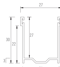
ART. 016702004 Guida in alluminio estruso con bordino e spazzolino 100279 30x27 mm
