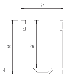
ART. 016702004 Guida in alluminio estruso senza bordino con spazzolino
