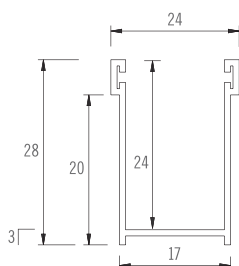
ART. 016502010 Guida in alluminio estruso con spazzolino 28x17 mm
