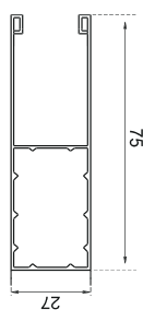
ART. Guida compatibile con mini cassonetto in alluminio 75x27 mm
