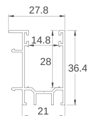
ART. ZAP 330 Profilo predisposizione con guida ad incasso per zanzariera 32,5x36,4 mm
