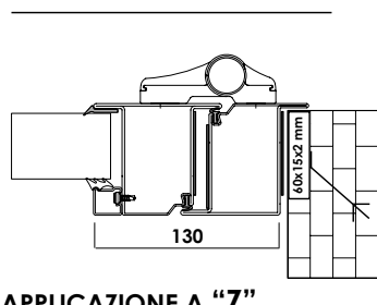
APPLICAZIONE A "Z"
