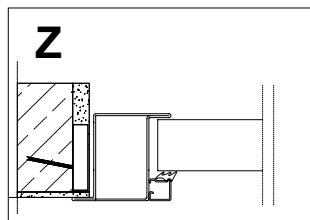
PROFILO "Z" su muro
