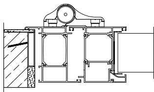
APPLICAZIONE A "Z"
