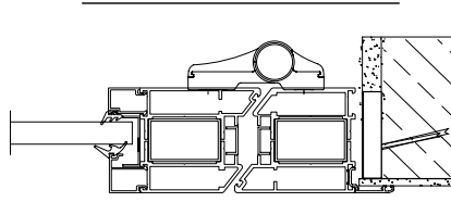
APPLICAZIONE A "T"
