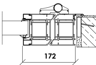
APPLICAZIONE AD "Z"
