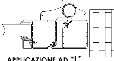
APPLICAZIONE AD "L"
