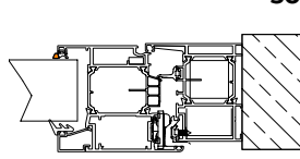
APPLICAZIONE AD "L"
