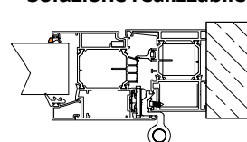
APPLICAZIONE AD "L"
