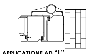
APPLICAZIONE AD "L"
