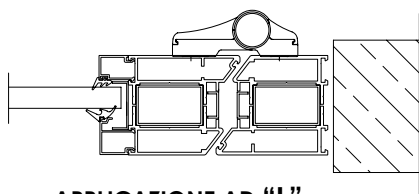
APPLICAZIONE AD "L"
