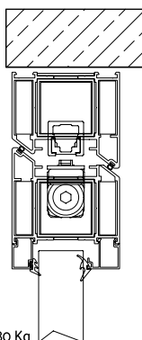
APPLICAZIONE A "T"
