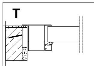
PROFILO "T" su muro
