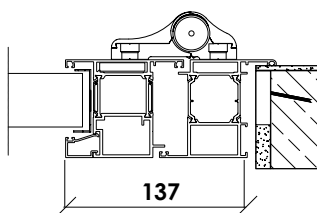
APPLICAZIONE A "Z"
