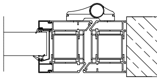
APPLICAZIONE AD "L"
