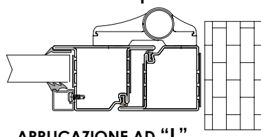
APPLICAZIONE AD "L"
