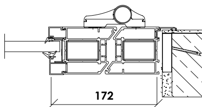
APPLICAZIONE A "Z"
