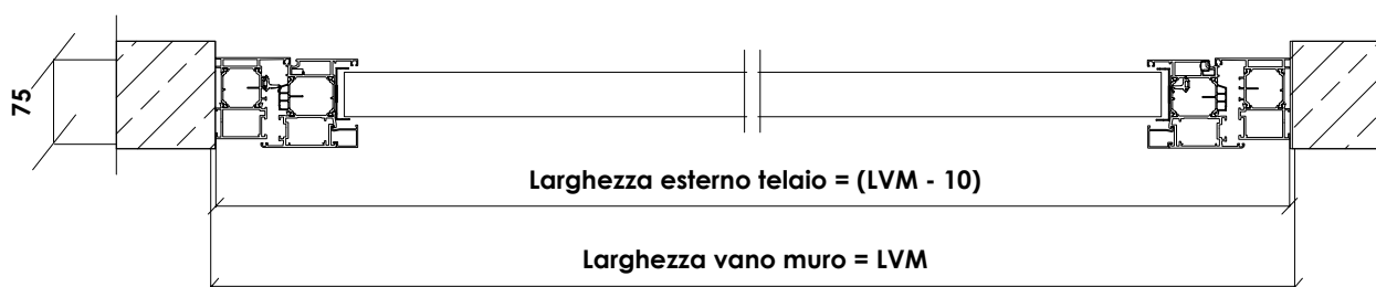
APPLICAZIONE AD "L"
