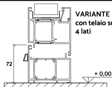
VARIANTE con soglia mobile basculante
