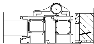
APPLICAZIONE A "T"
