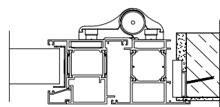
APPLICAZIONE A "T"
