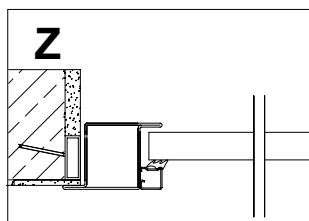
PROFILO "Z" su muro
