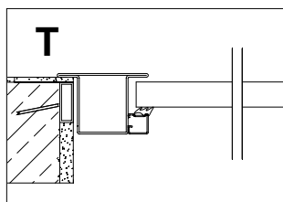
PROFILO "T" su muro
