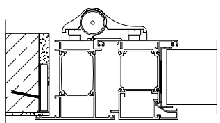
APPLICAZIONE A "T"
