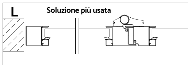
PROFILO "L" su muro
