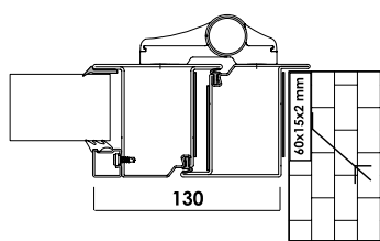
APPLICAZIONE A "Z"
