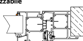
APPLICAZIONE A "Z"
