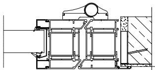
APPLICAZIONE AD "T"
