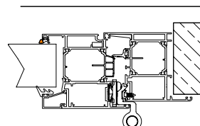
APPLICAZIONE A "Z"
