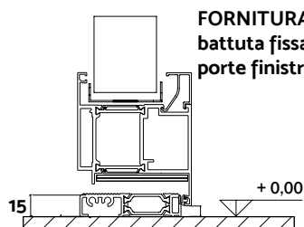
APPLICAZIONE A "T"
