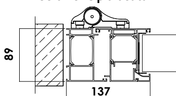
APPLICAZIONE AD "L"
