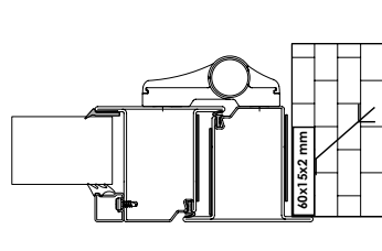
APPLICAZIONE A "T"
