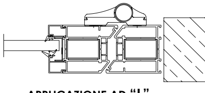
APPLICAZIONE AD "L"
