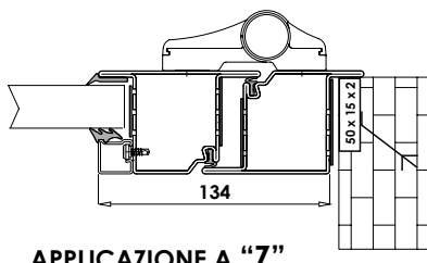
APPLICAZIONE A "Z"
