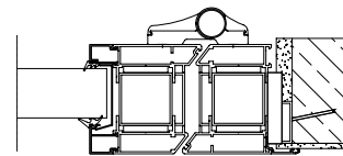
APPLICAZIONE A "T"
